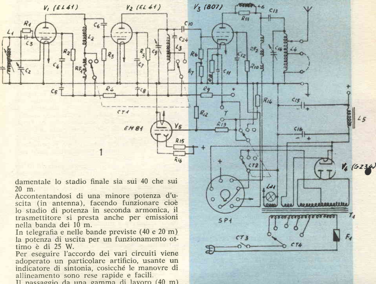
SCHEMA ELETTRICO DEL TRASMETTITORE
